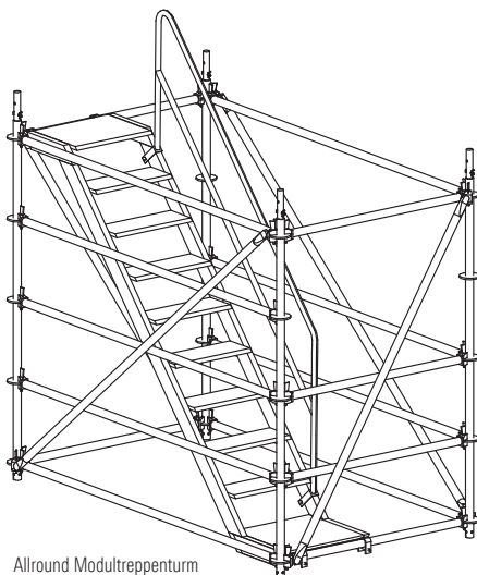
Allround Modultreppenturm 2,20 m hoch
