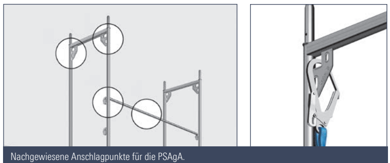
Nachgewiesene Anschlagpunkte für die PSAgA.
