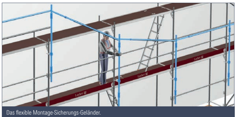
I-Geländer – systemintegriert.
